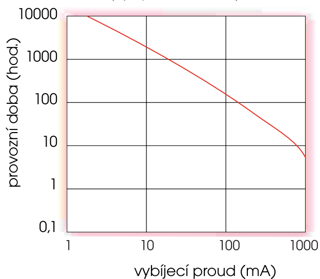
Trvalý vybíjecí proud (vybiteno do 0,9 V)
