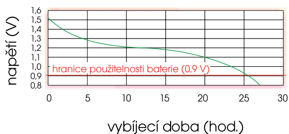
svítilna 2,2Ω - 4 min./hod.- 8 hod./den
