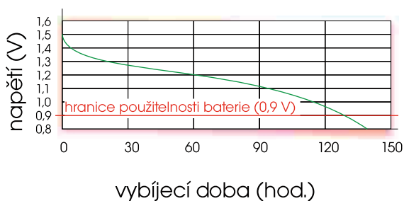
rádio 10Ω - 4 hod./den
