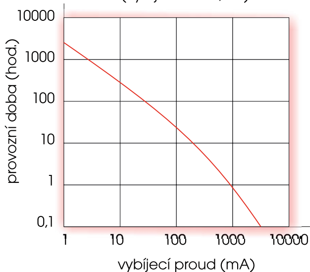
Trvalý vybíjecí proud (vybitý do 0,9 V)
