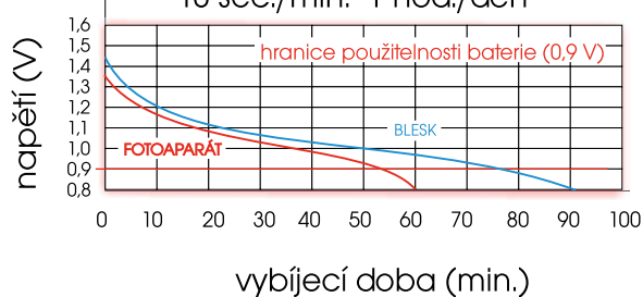
digitální fotoaparát (I = 1 A) - 10 sec./min.- 1 hod./den
