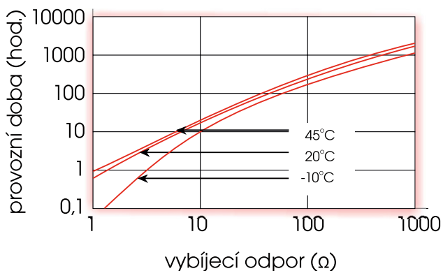
Vliv okolní teploty na vybití baterie (vybitý do 0,9 V)
